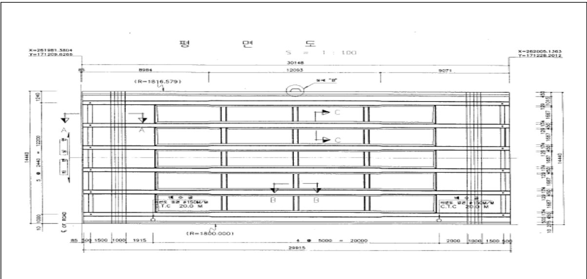
<그림 6.7>범안대교(범물방향) 상부 일반도(1)
